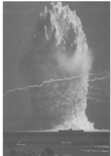
Abb. 29: Unterseeischer Atomtest der USA in Eniwetok Lagune, Südpazifik, 1958
