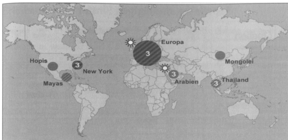
Abb. 45: Voraussagen zur dreitägigen Finsternis weltweit
