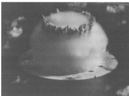
Abb. 32: US-Atombombentest, Juli 1946
