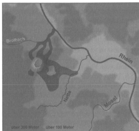
Abb. 10: Der Laacher-See-Vulkan
