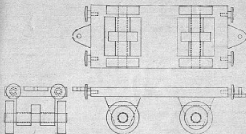
Eisenbahnplattformwagen
