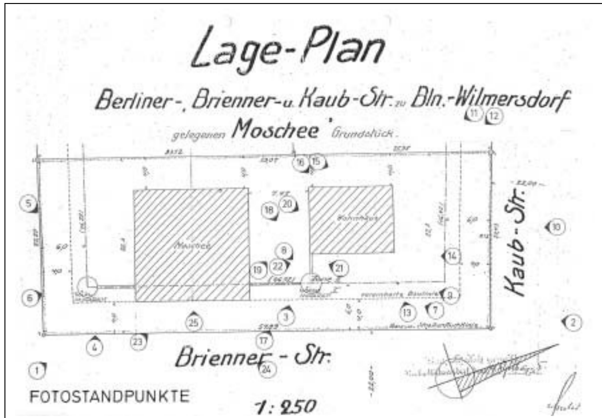
Original-Lageplan der Berliner Moschee mit späteren Nachträgen
