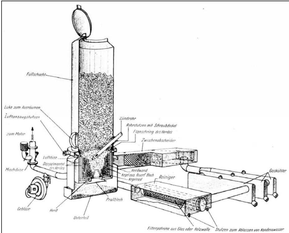
Abb. 133: Funktionsweise einer Ostmark Generatorgas-Anlage.
