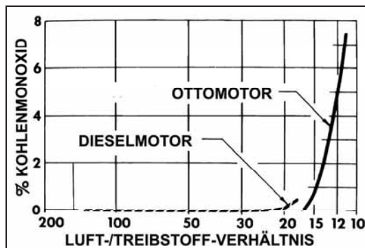
Abb. 128: Kohlenmonoxid-Gehalt von Abgasen aus Otto- und Dieselmotoren in Abhängigkeit von der Motorlast (Luft-/Treibstoff-Verhältnis)
