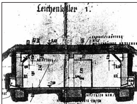
Abb. 122: Querschnitt des Leichenkellers 1 von Krematorium II. Der Keller ist innen 7 m breit, die Tür etwa 2 m. 212
