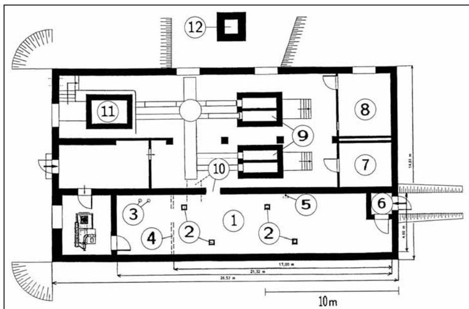
Abb. 107: Grundriss des Krematoriums I im Lager Auschwitz I/Stammlager heute, nach den nachträglichen Manipulationen.
