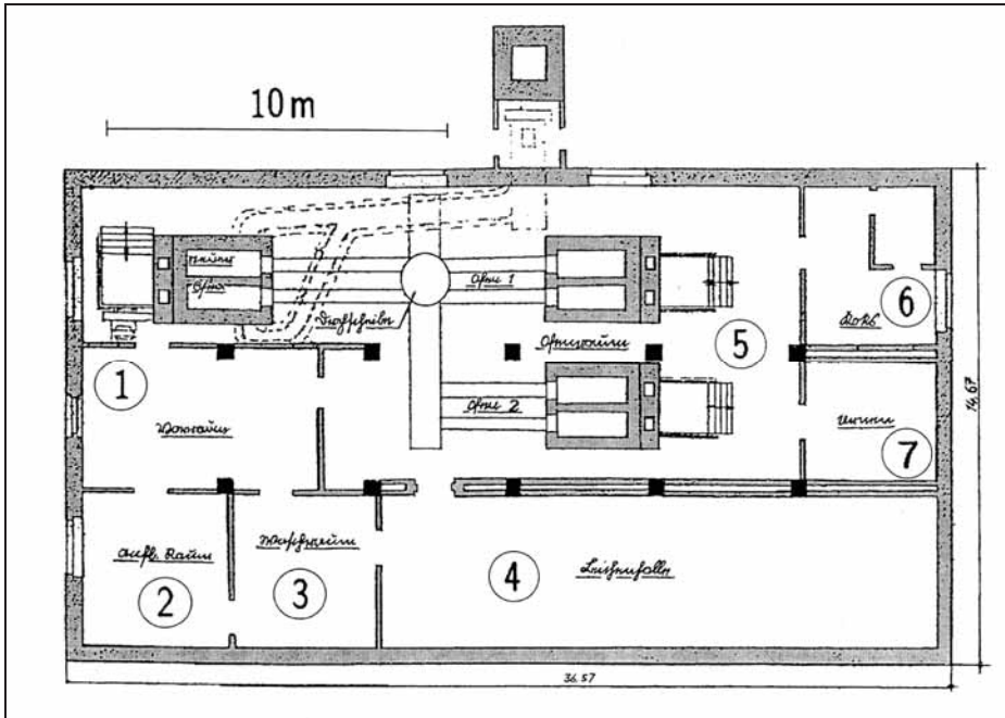
Abb. 104: Grundriss des Krematoriums I im Lager Auschwitz I/Stammlager im ursprünglichen Planungszustand. Die Leichenhalle soll später angeblich als Gaskammer benutzt worden sein. 1: Vorraum; 2: Aufbahrungsraum; 3: Waschraum; 4: Leichenhalle; 5: Ofenraum; 6: Koks; 7: Urnen
