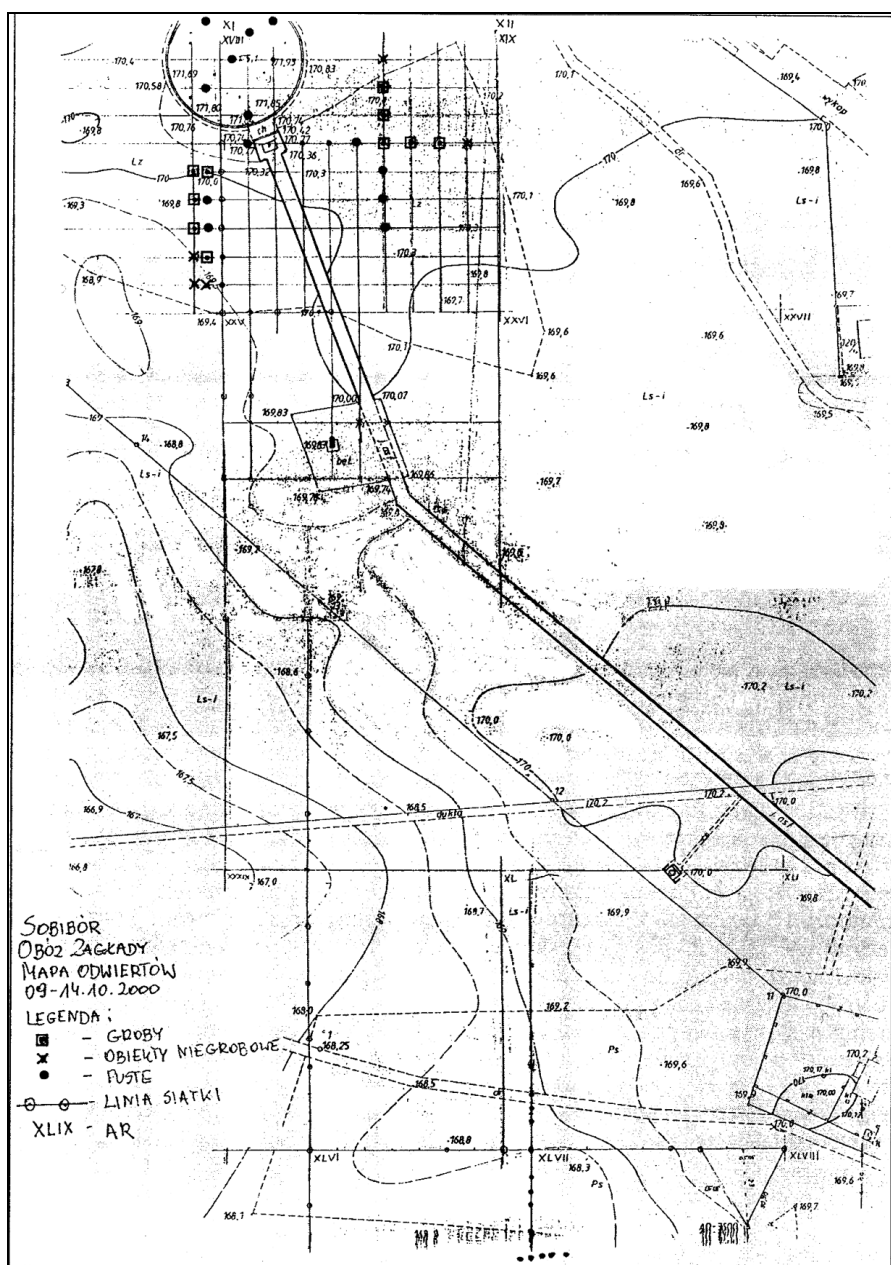
Dokument 6: Karte der Gegend um das vormaligen Lager III mit Teilen des archäologischen Netzwerkes. Quelle: A. Kola, aaO. (Anm. 326), S. 92.
