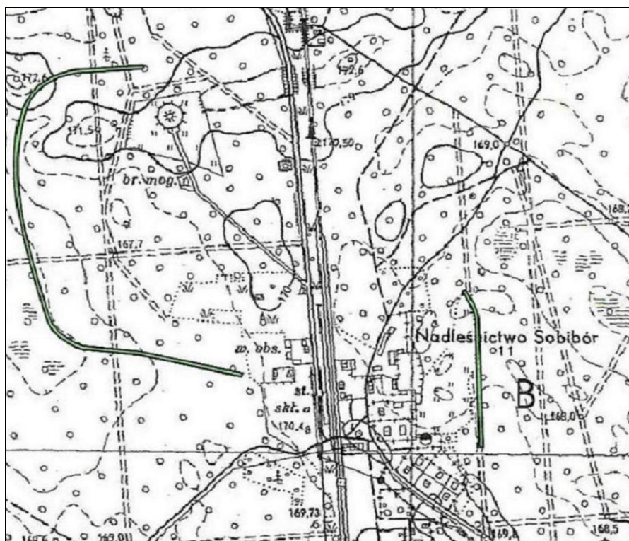
Dokument 4: Eine moderne topographische Karte der Sobibór-Gegend. Die Gegend mit dem Denkmal befindet sich oben links. Quelle:
