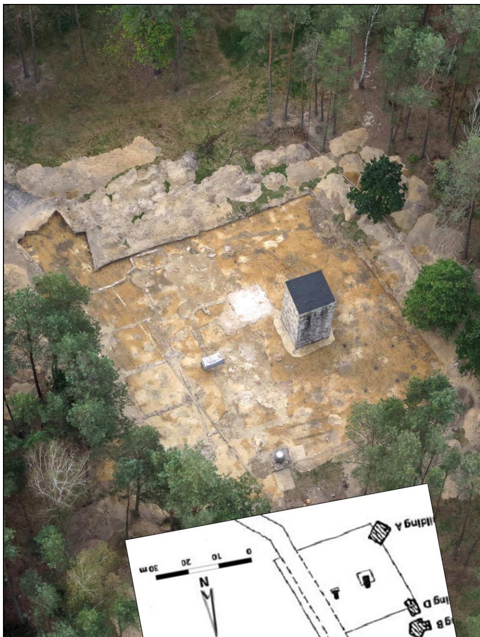
Illustration 1: Luftbild aus dem Jahre 2014 von Ausgrabungen um das alte Denkmal auf dem Gebiet des vormaligen Lagers Sobibor.
