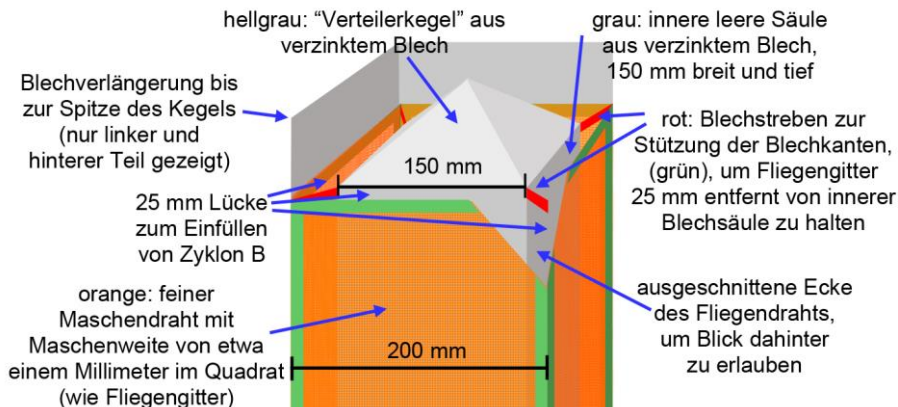
Abbildung 25: Schemazeichnung des oberen Teils der innersten Säule der Einwurfvorrichtung, wie sie anfangs von Kula am 11.6.1945 beschrieben wurde. (Rudolf 2017b, S. 153).
